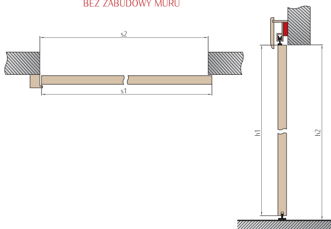
SYSTEM PRZESUWNY BEZ ZABUDOWY MURU
