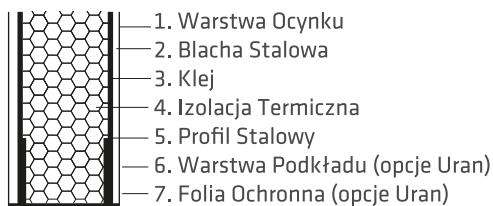
Przekrój pionowy
